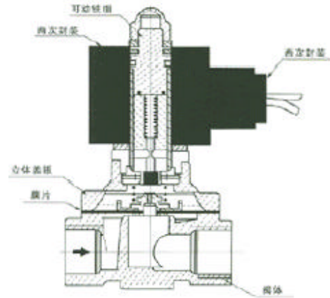
外形尺寸、内部结构图
