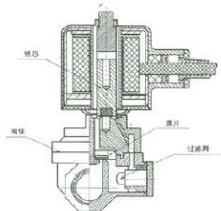
外形尺寸、内部结构图
